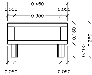
VISTA LATERAL ESC.: 1:15
