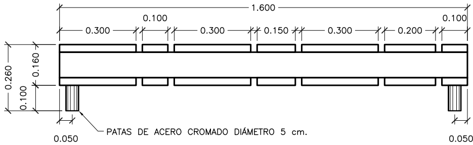
VISTA FRONTAL ESC.: 1:15
