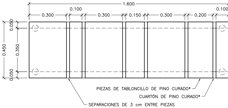
PLANTA ESC.: 1:15
